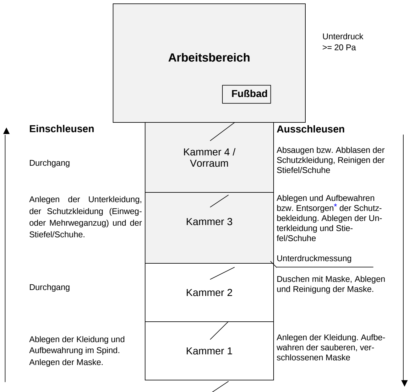
Abb. 1 Personenschleuse (Prinzipskizze)
